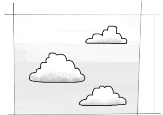
Stapelwolken Cumulus
