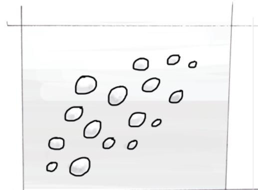
Schaapjeswolken Altocumulus
